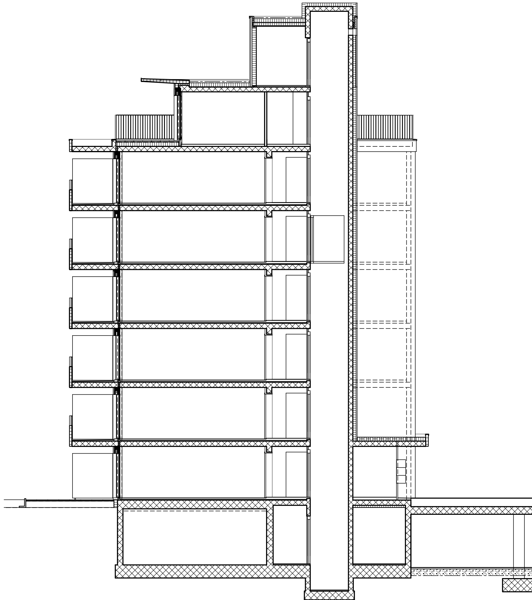
HAUS 4 SCHNITT 1:100
